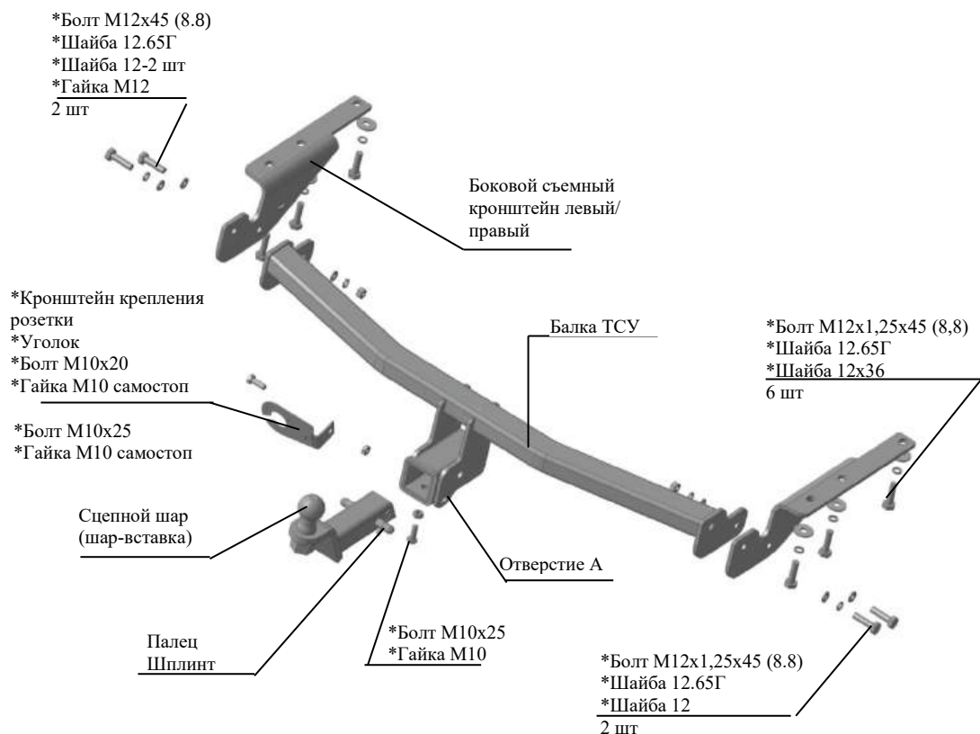
Рис.1 Тягово-сцепное устройство 7835.
